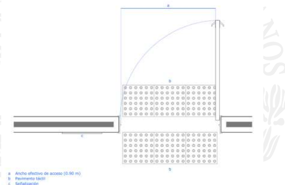
Figura 18 - Detalle de puertas
