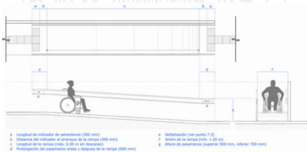
Figura 8 - Detalle de rampa
