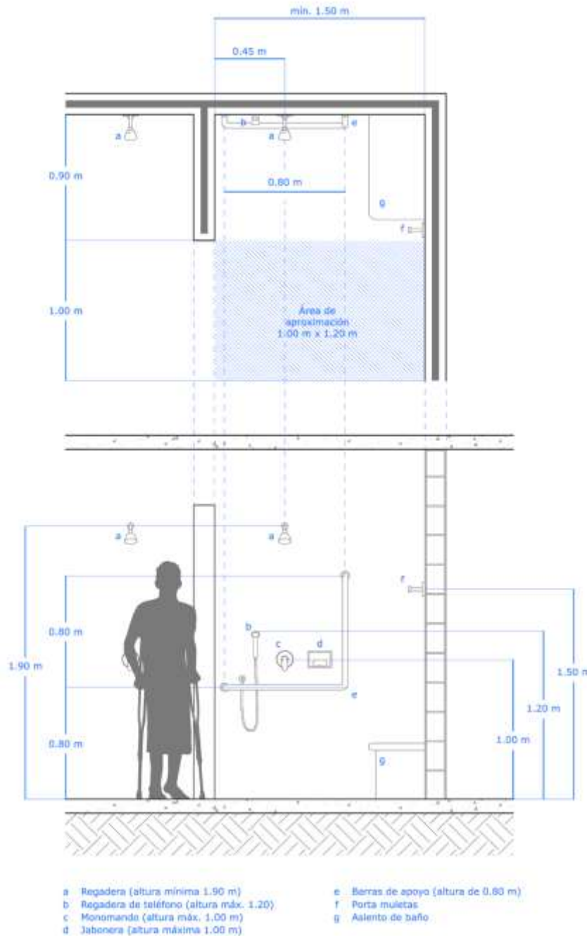
Figura 24 - Dimensionamiento de regaderas
