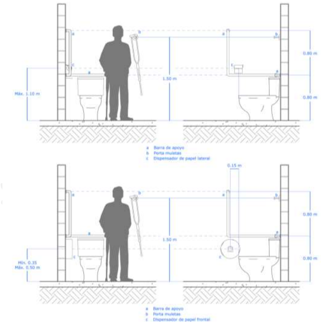
Figura 25 - Accesorios
